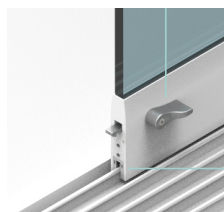
Apertura interna con maniglia standard (Fly o Quadra) e pedale 75€
